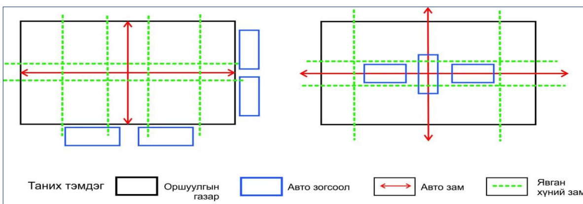
Зураг 6. Авто зогсоолын төлөвлөлтийг хийх загвар зураг
